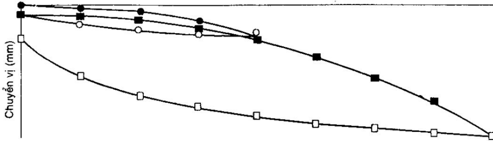
Hình B.1 – Biểu đồ quan hệ tải trọng – chuyển vị
