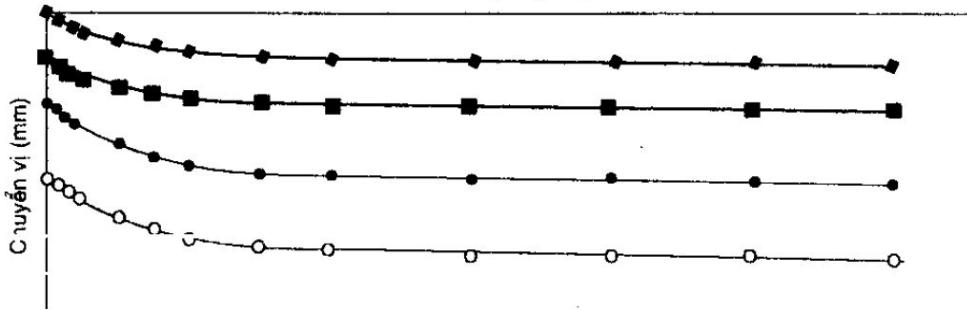
Hình B.2 – Biểu đồ quan hệ chuyển vị - thời gian
