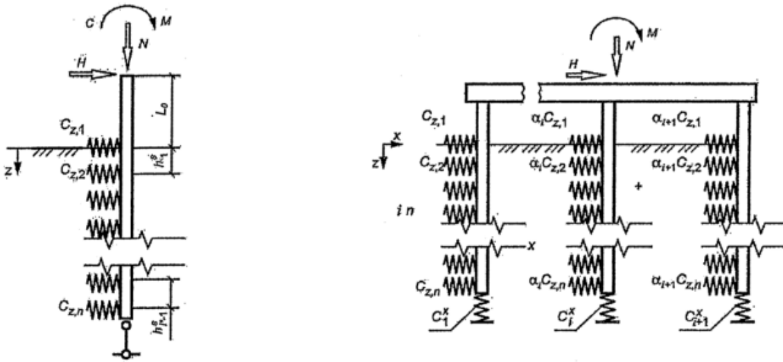
a) Sơ đồ tính toán cọc đơn
