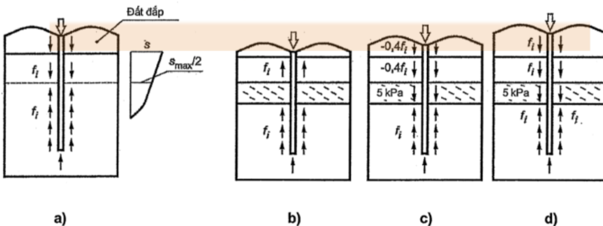
a) Trường hợp tổng quát; b) Khi có lớp đất yếu mỏng và chiều cao đắp < 2 m; c) Khi có lớp đất yếu mỏng và chiều cao đắp từ 2 m đến 5 m; d) Khi có lớp đất yếu và chiều cao đắp > 5 m
