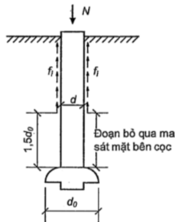
Hình 2 – Sơ đồ tính toán sức kháng đơn vị trên mặt bên thân của cọc mũi mở rộng trong đất cát
