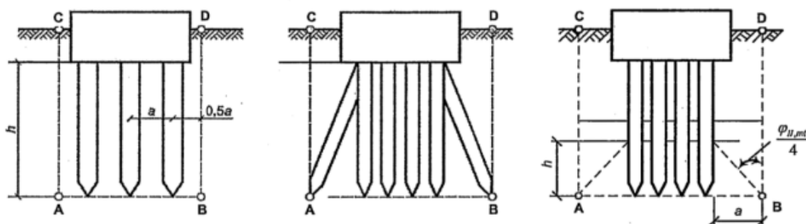
a) Khi chỉ có các cọc thẳng đứng
